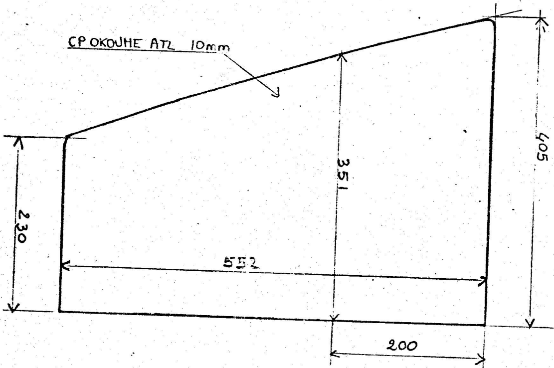
FOND SUPERIEUR
